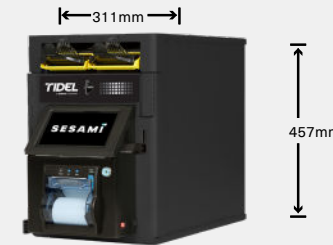
Tidel S4 XL
